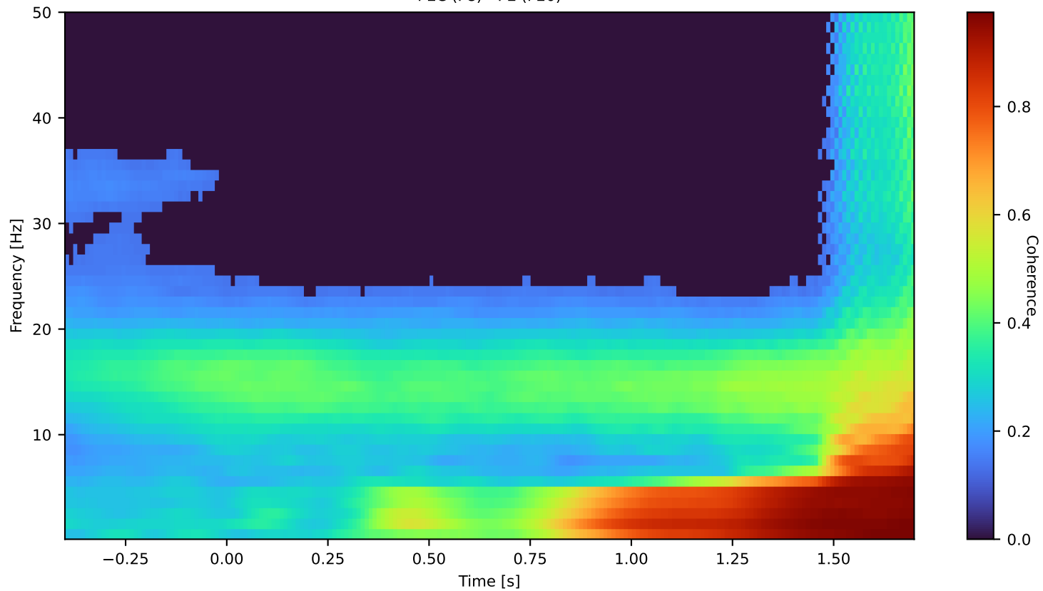
PEC (P8) - PE (P20)
